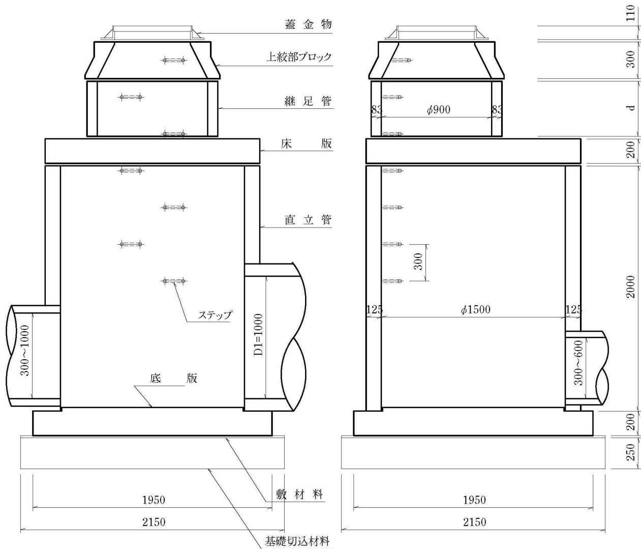
正面図
