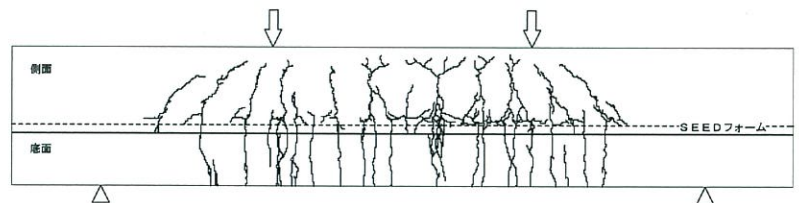
「SEEDフォーム(O)」を引張縁に配置したRC部材の破壊状況
